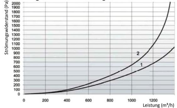
Strömungskennlinien E-Flex - Länge 4 m
